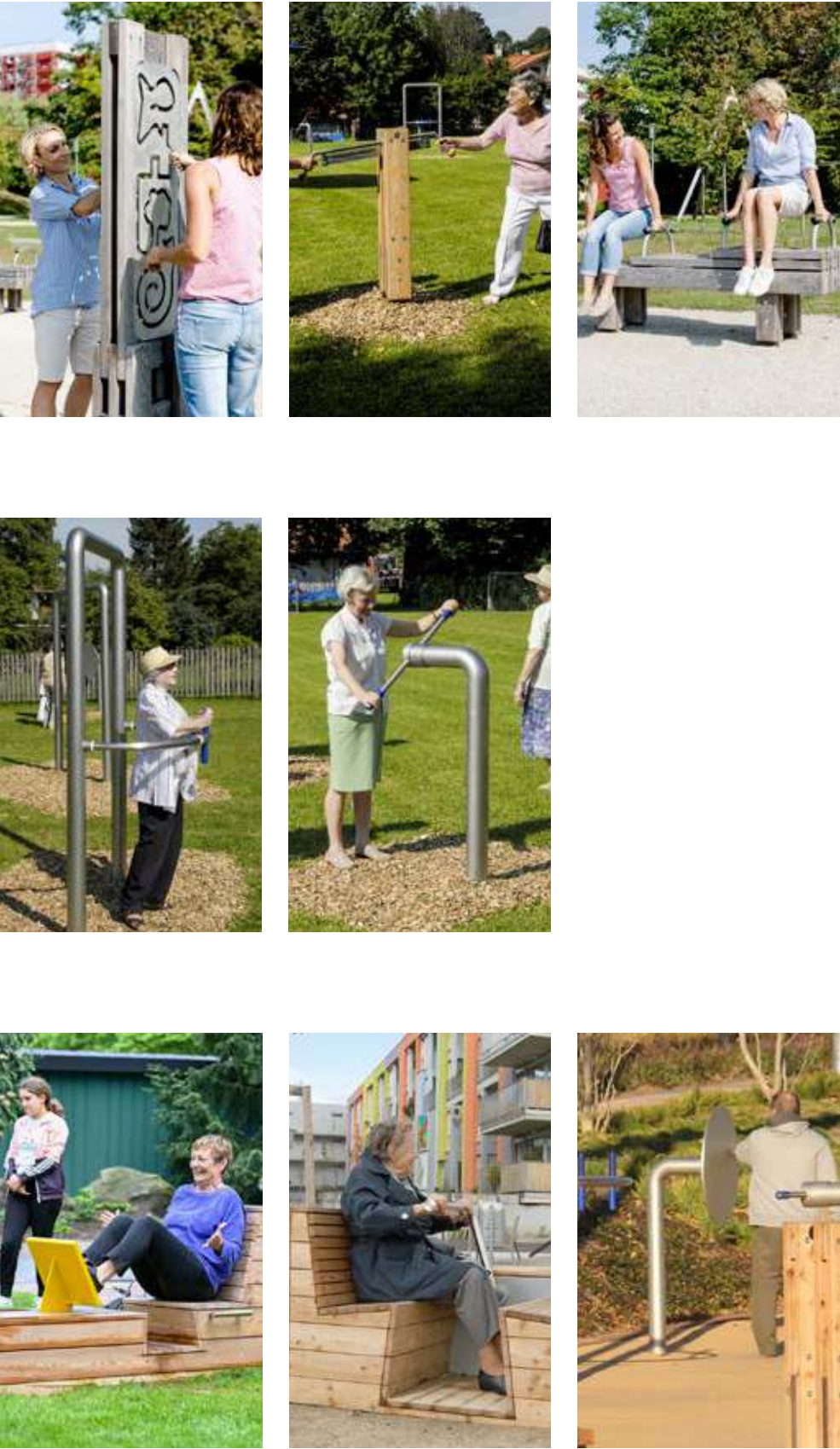
TRILHO DE CURVA • SERRA • BANCO DE DEGRAUS • ARCO DE VIRAGEM • BARRA DE VIRAGEM • PRENSA DE PERNAS • MÁQUINA DE REMO • DISCO • TURNING PLATE
